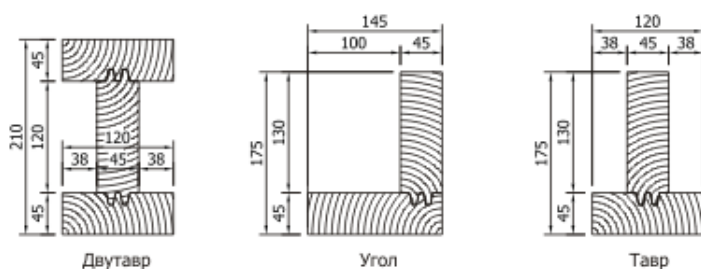
рис.1 элементы каркаса
